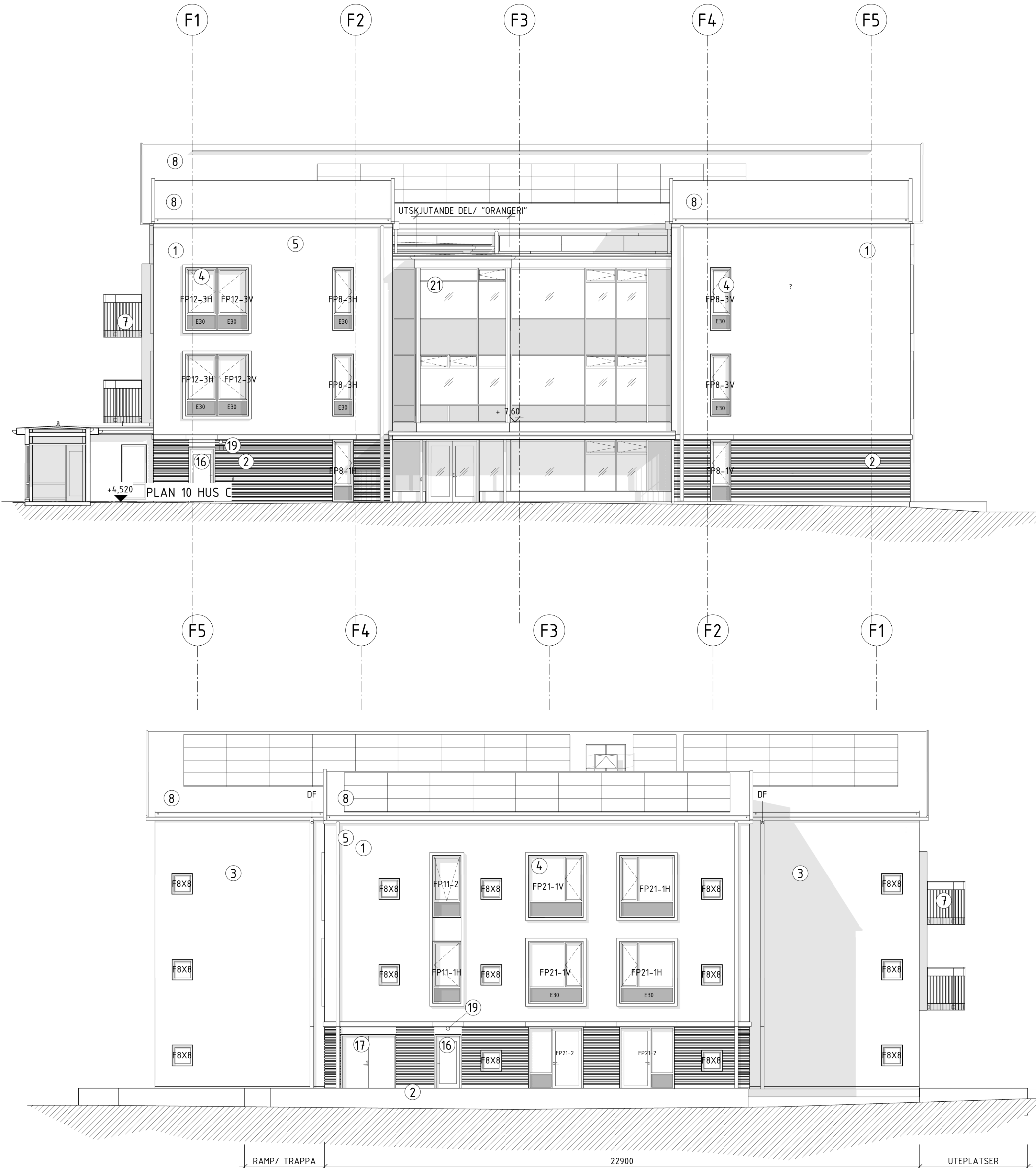
A-40-3-1030 VÄSTER 1 : 100
