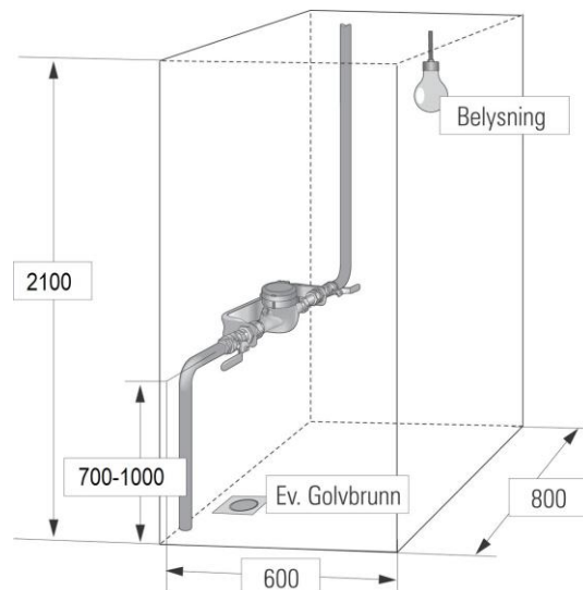
Fig. 1. För att komma åt vattenmätaren för avläsning eller service måste det finnas ett fritt utrymme runt mätaren enligt denna figur. Alla mått i mm.
